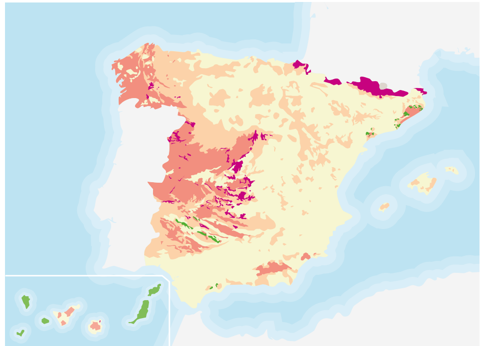
Mapa del potencial de radón en España. Enero 2017
